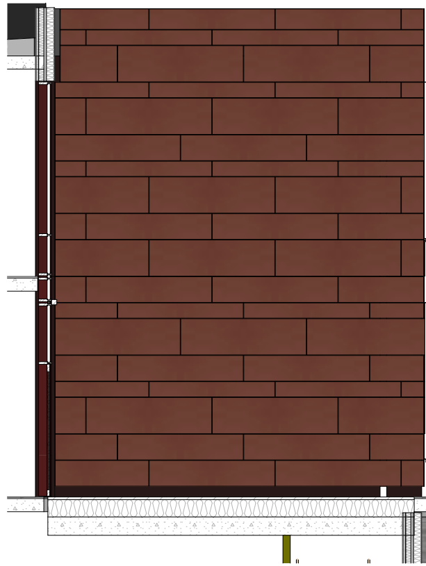
Fasade øst akse 9
